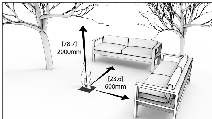
1. 户外安装
