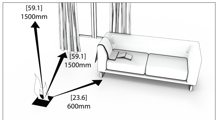
Sicherheitsabstände im Innenbereich
