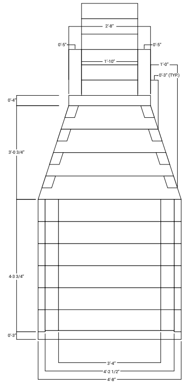
FIGURE 1.4 48" RUMFORD
