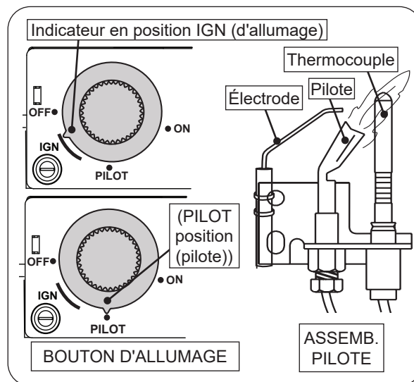
Fig. 58-1 Éclairage pilote
