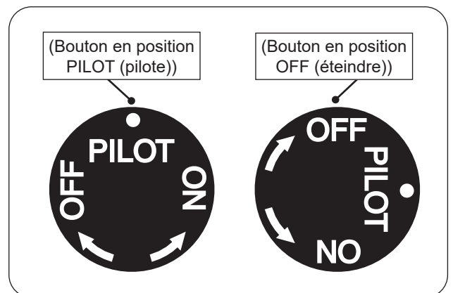
Fig. 62-2 Arrêt manuel
