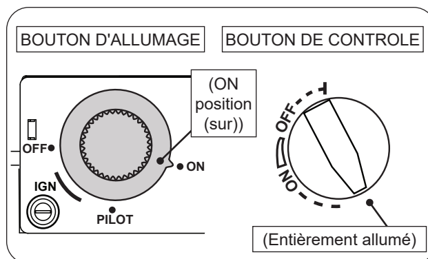
Fig. 59-1 Éclairage manuel
