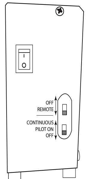
Fig. 16 Module Switches
