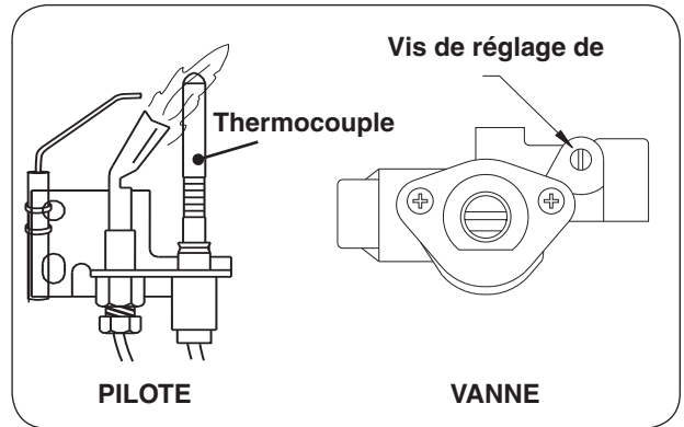
Fig. 24-1 Détail réglage de la veilleuse
