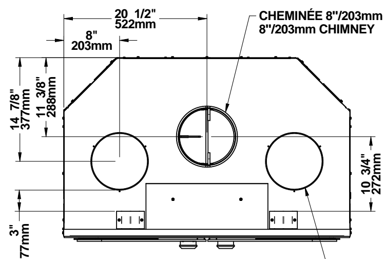
ENS. DIST. PAR GRAVITÉ 8"/203mm (2) 8"/203mm GRAVITY AIR KIT (2)
